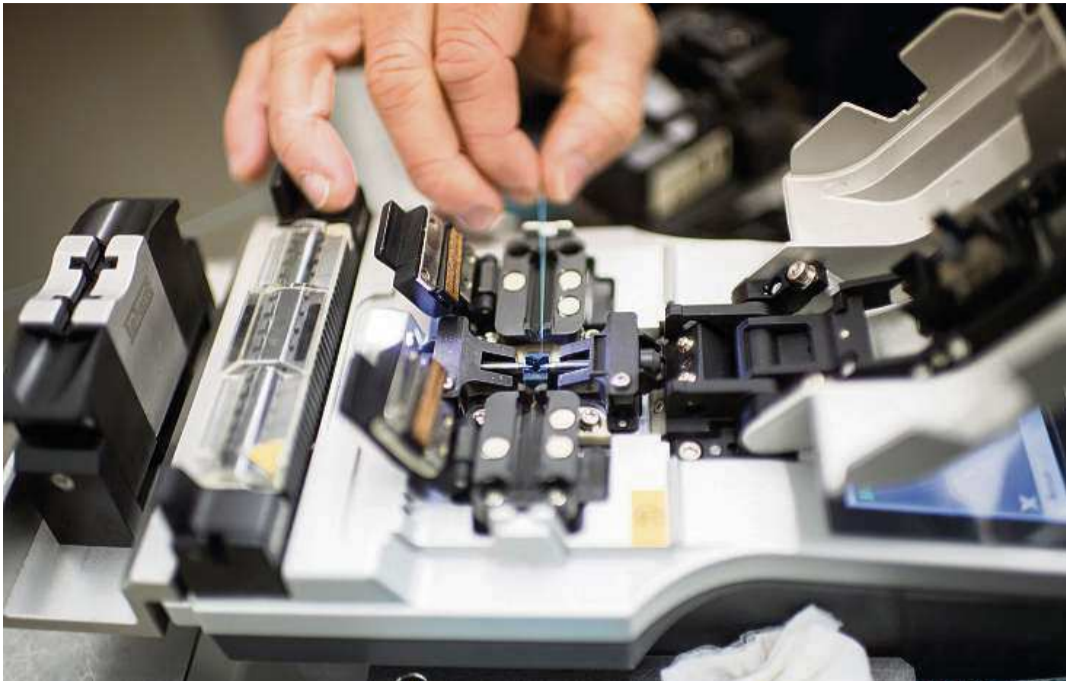
Verbindung von Lichtwellenleitern, sogenanntes «Spleissen» von Glasfasern.
